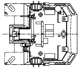
Topdeck
